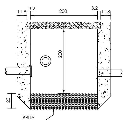
CORTE - B B' CAIXA DE PASSAGEM SUBTERRÂNEA
