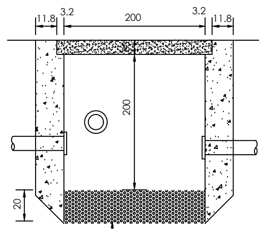
CORTE - B B' CAIXA DE PASSAGEM SUBTERRÂNEA
