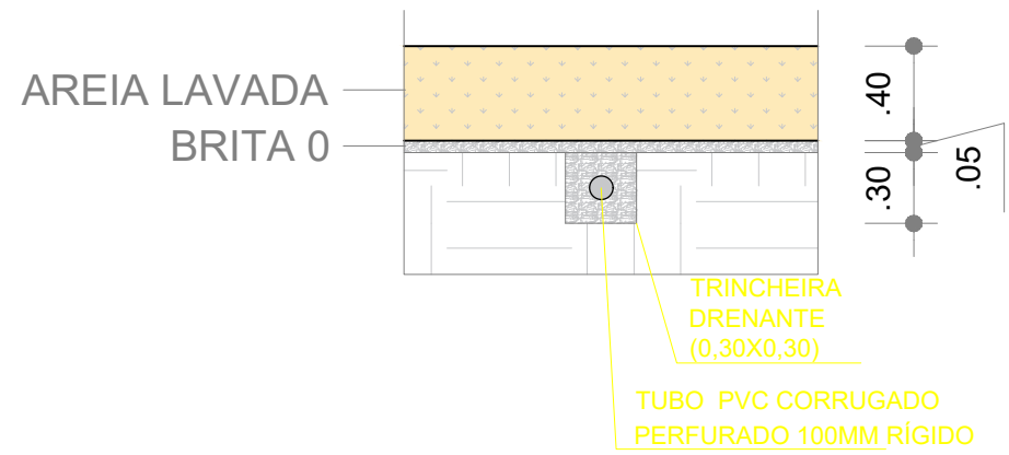
DETALHA TRINCHEIRA DRENANTE
