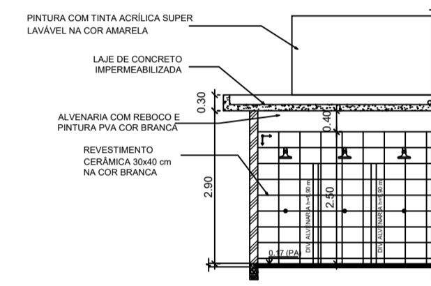
VESTIÁRIO: VISTA C ESC 1:100
