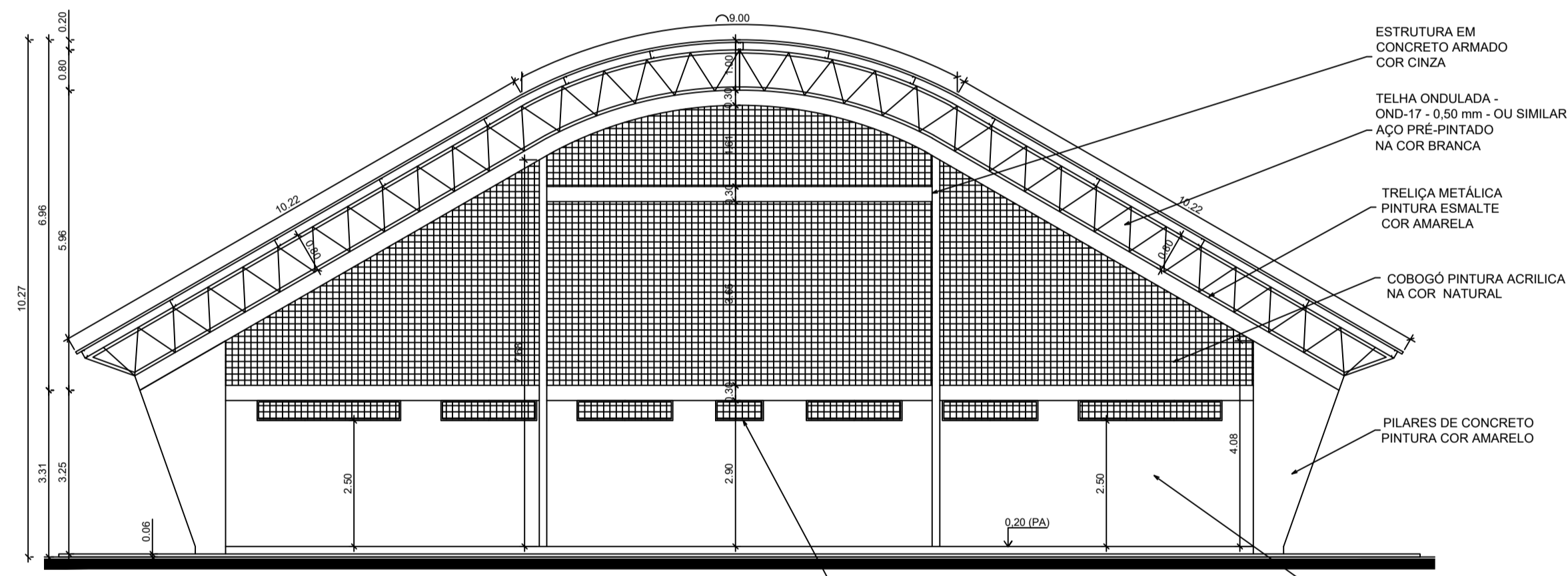
FACHADA 03 ESC 1:100
