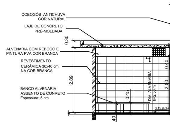
VESTIÁRIO: VISTA B ESC 1:100
