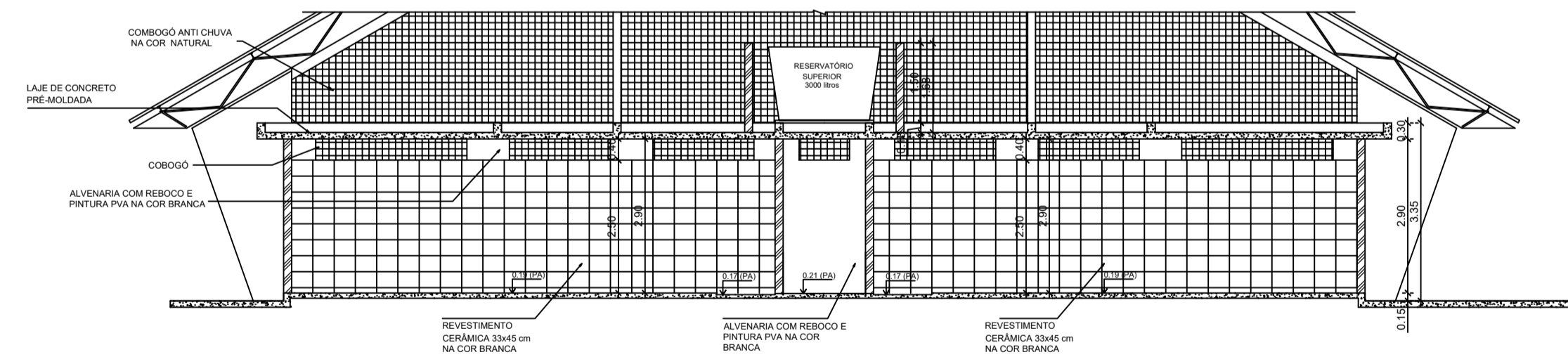
VESTIÁRIO - CORTE DD ESC 1:100
