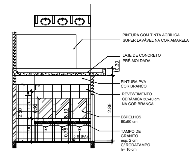
VESTIÁRIO: VISTA A ESC 1:100
