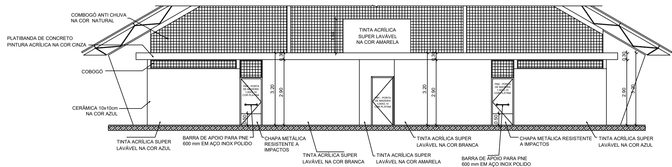
VESTIÁRIO: VISTA E - FACHADA FRONTAL ESC 1:100
