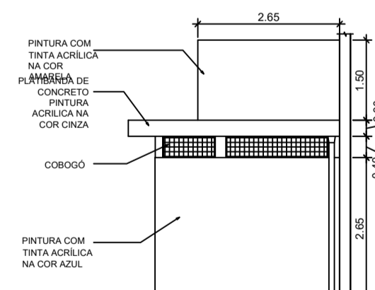
VESTIÁRIO: VISTA F - FACHADA LATERAL ESC 1:100
