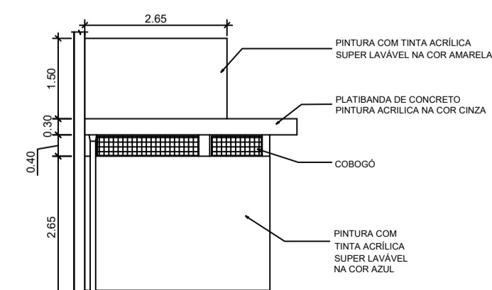
VESTIÁRIO: VISTA G - FACHADA LATERAL ESC 1:100
