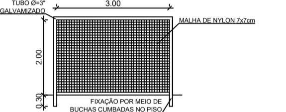
BALIZA FUTEBOL VISTA FRONTAL ESC 1:100
