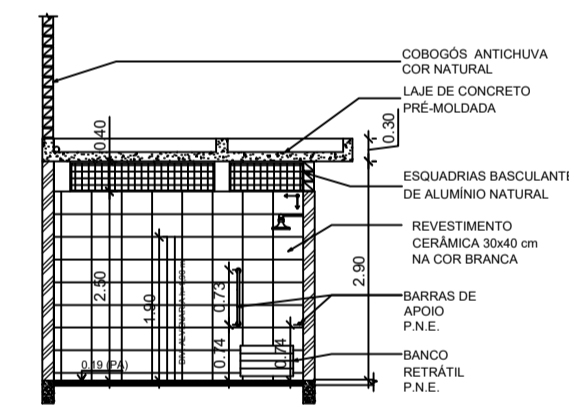
VESTIÁRIO: VISTA D ESC 1:100
