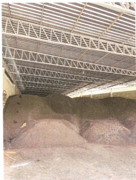
FOTO 1: Execução de cobertura metálica
