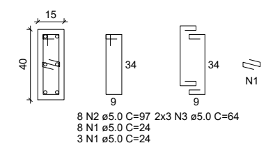
SEÇÃO A-A ESC 1:25
